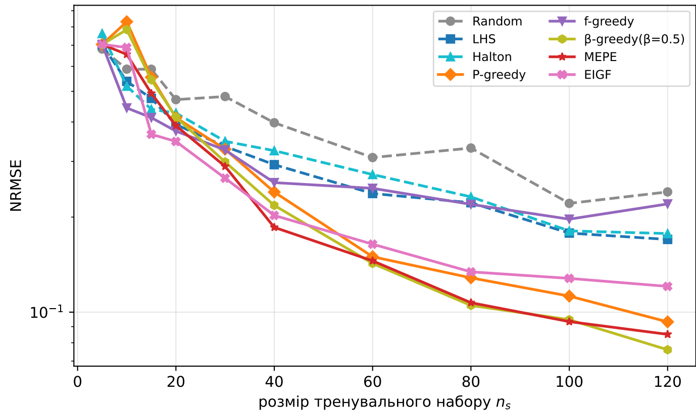
Збіжність помилки сурогата для q
